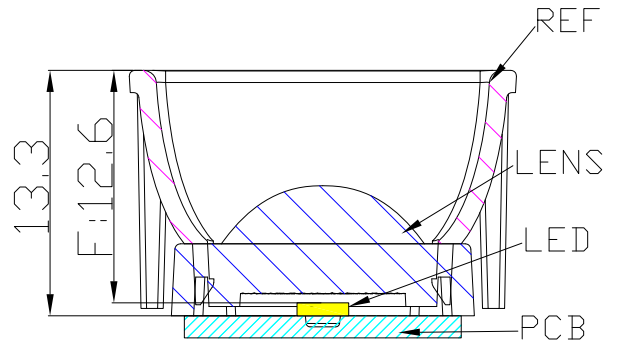
光学装配示意图
